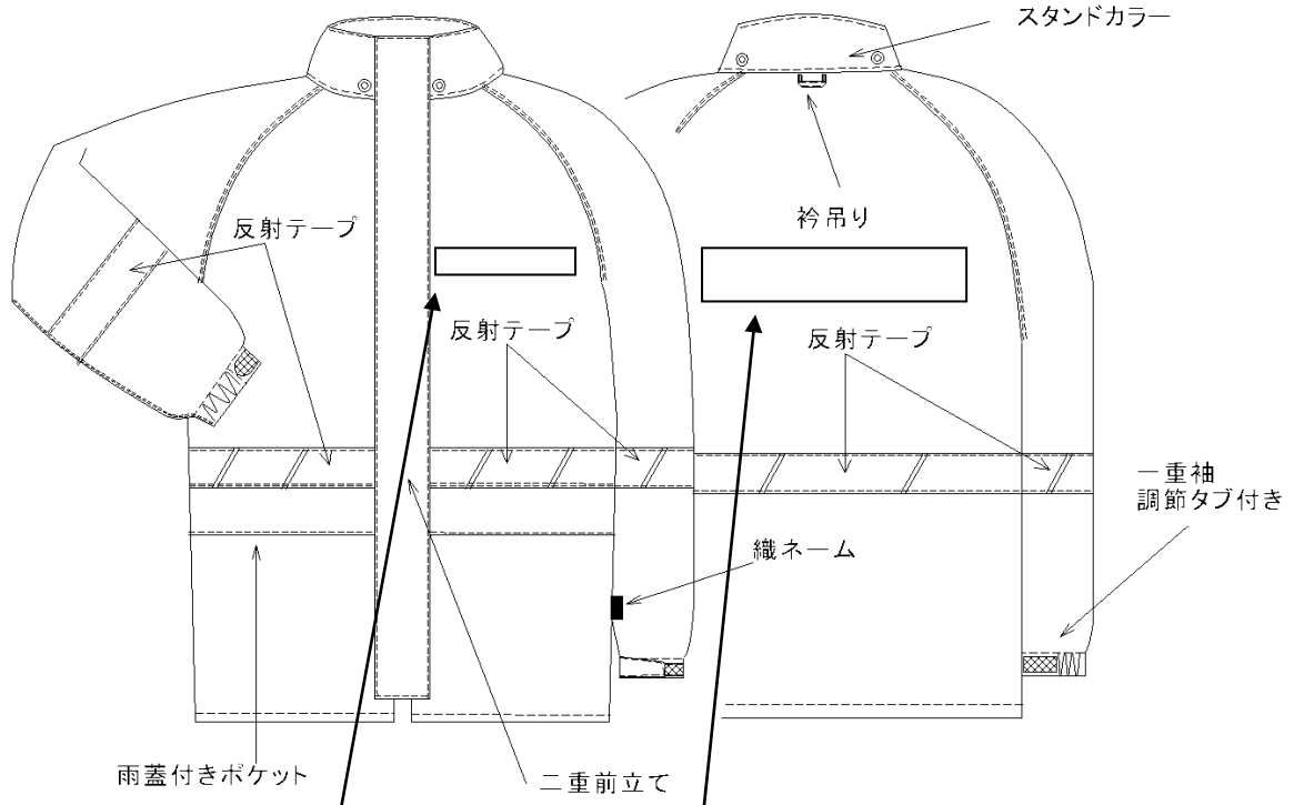
上衣全体図
